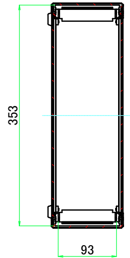
A-A ( 1 : 6 )
