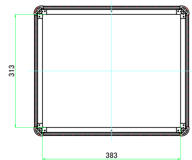
C-C ( 1 : 6 )
